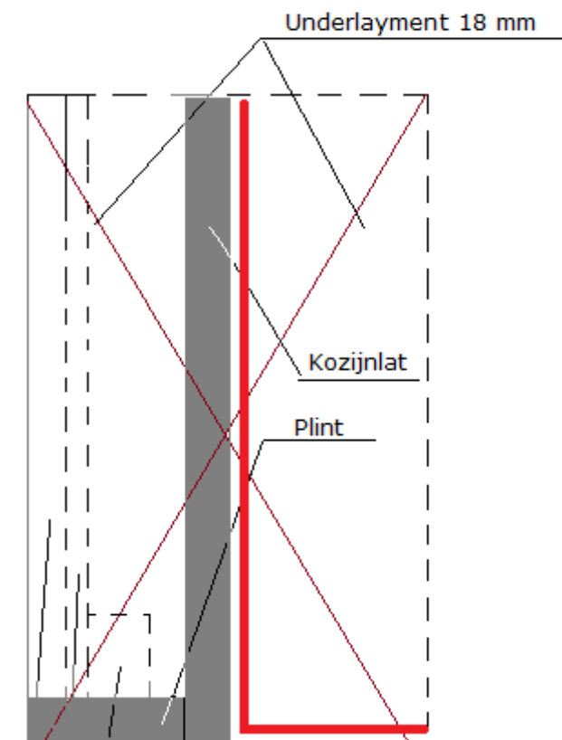
Detail vooraanzicht
